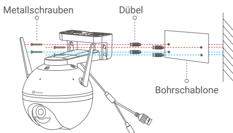
Abb. 1 Wandmontage
